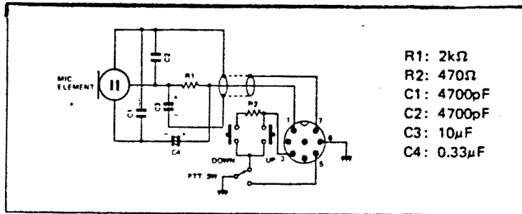
Schema elettrico dello HM-36
